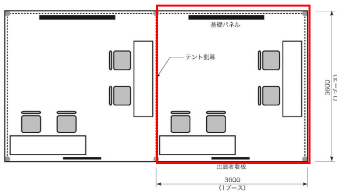
平面図
