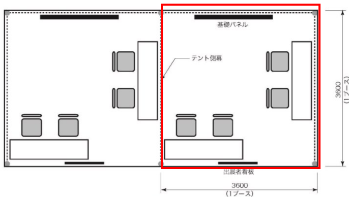
平面図
