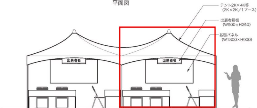
正面図
