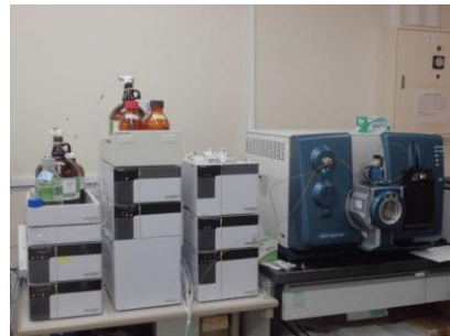
■液体クロマトグラフ質量分析装置（LC-MS/MS）による分析
