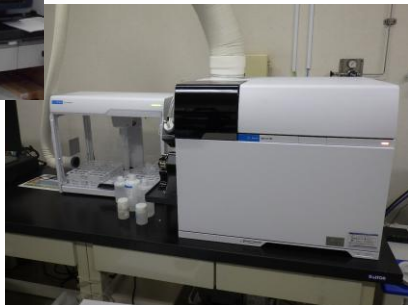
■誘導結合プラズマ質量分析装置（ICP-MS）による分析
